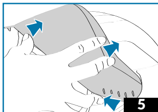
5 - Premere simultaneamente i pulsanti "L" e "R", poi spingere con le altre dita da ambo i lati, sotto la visiera, per liberarla verso il retro del casco. Trattenere la visiera alla fine dell'operazione.
