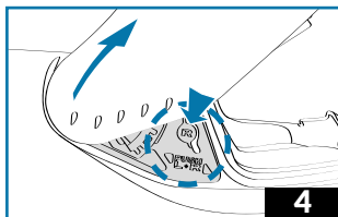
4 - Su ognuno dei supporti meccanici laterali, individuare, su ambo i lati della visiera, un pulsante con l'iscrizione "R" sul lato destro e con l'iscrizione "L" su quello sinistro.
