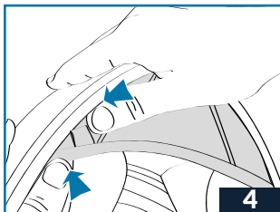
4 - Exercer des pressions de part et d'autre de la bavette pour s'assurer de sa bonne fixation.
